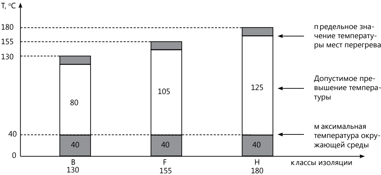
Рис. 7.1. Классы изоляции
