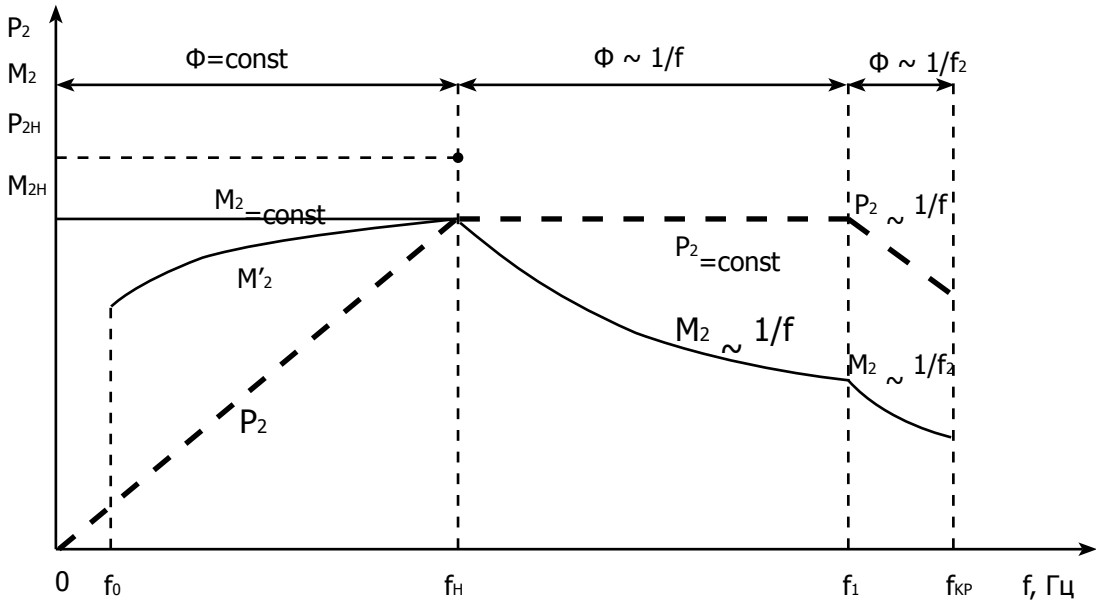
Рис. 2.1. Нагрузочные характеристики
