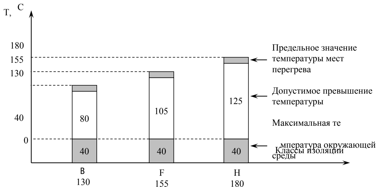
Рис. 5.1. Классы изоляции
