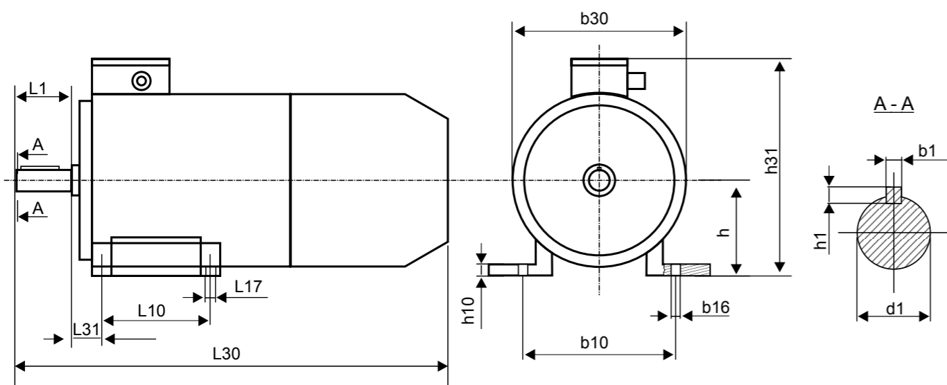
Рис. 14.1. Габаритные и установочно-присоединительные размеры (IM1001)
