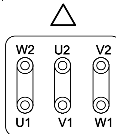
Рис. 15.1. Схема соединения «треугольник»
