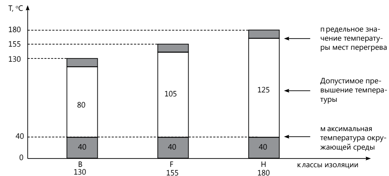
Рис. 7.1. Классы изоляции
