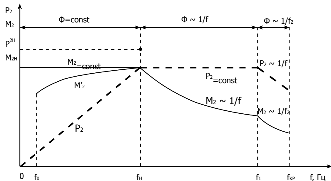
Рис. 2.1. Нагрузочные характеристики
