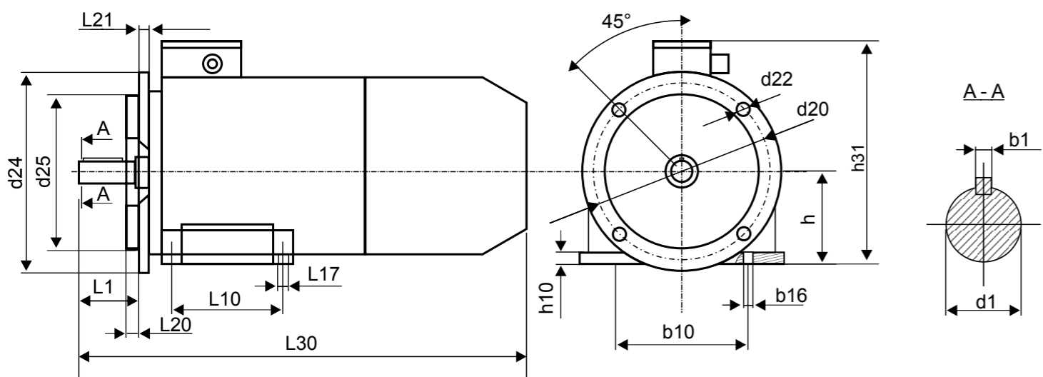
Рис. 14.2. Габаритные и установочно-присоединительные размеры (IM2001)
